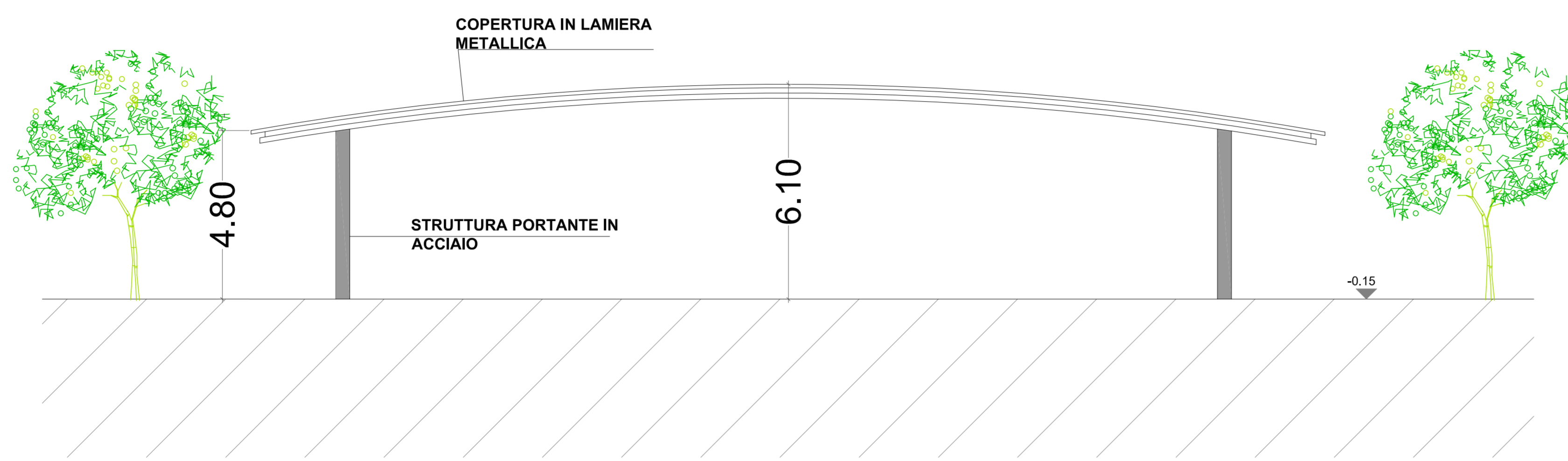
SEZIONE G - G
